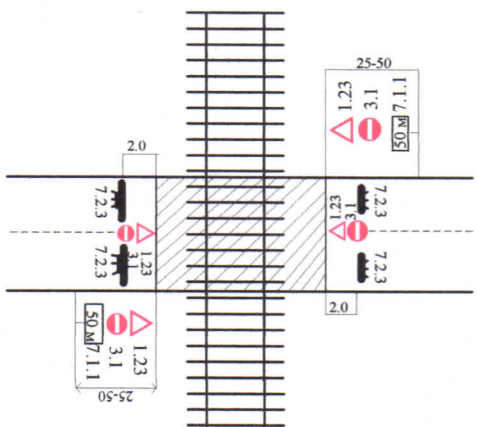
Схема ограждения места производства работ при ремонте железнодорожного переезда 883 км, пересекаемого ул. Опшманской на ст. Опшманы
